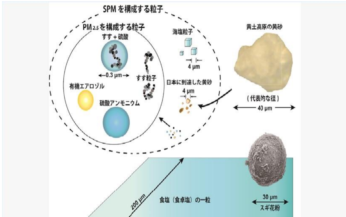
【図1】SPM, PM2.5を構成する粒子の大きさ
