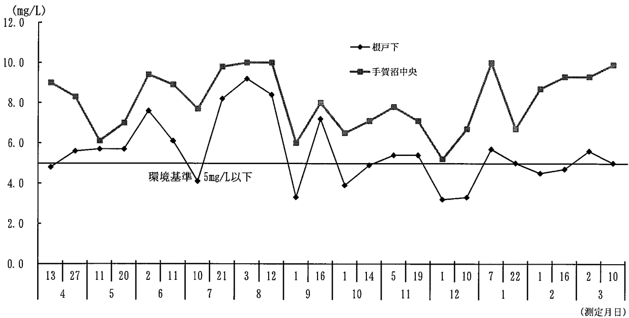
図1-8 手賀沼のCODの月別変化(平成27年度)
