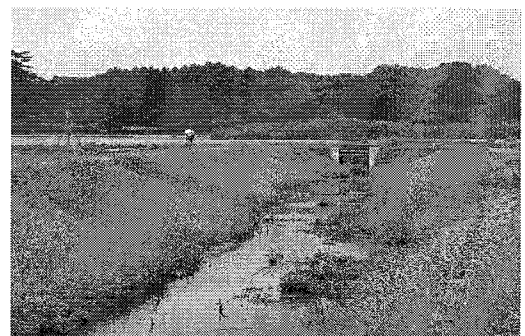
図 2-5 多自然型護岸
