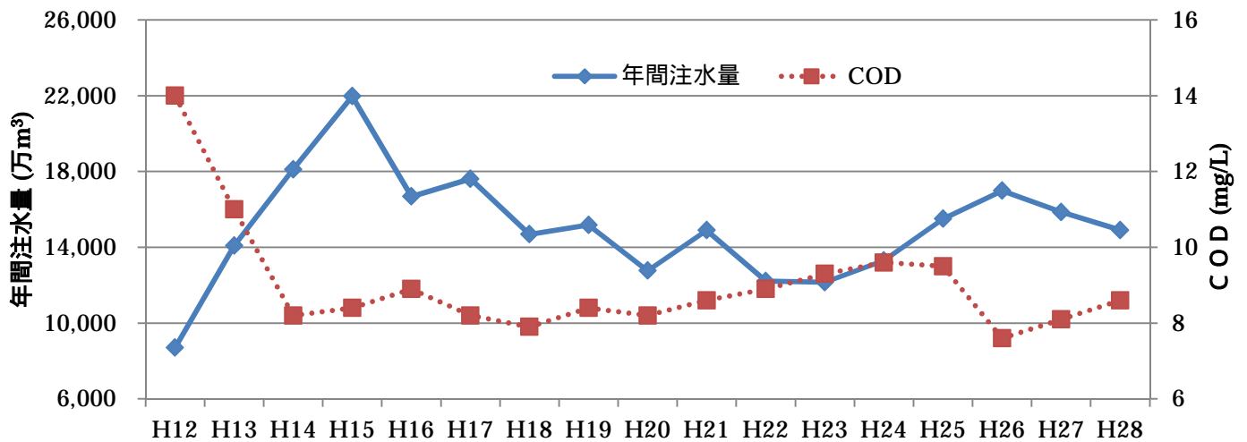
図1 - 13 北千葉導水年間注水量およびCOD
