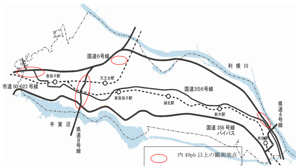
図1-10 窒素酸化物濃度等濃度線図(令和3(2021)年1月調査)単位:ppb*
