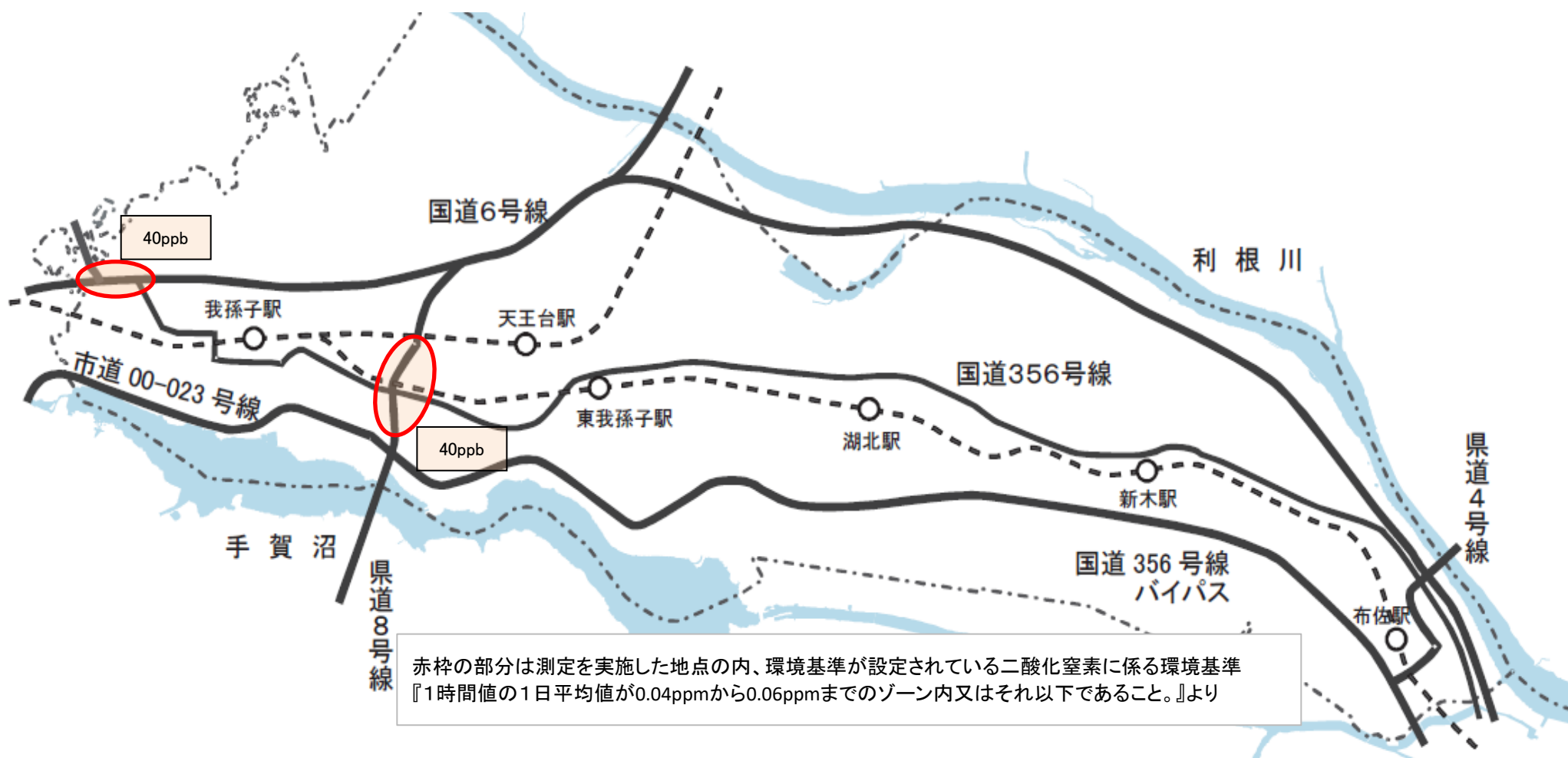
図3-5 窒素酸化物等濃度線図(概略図)
