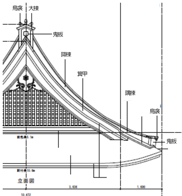
↑お配りした図面の抜粋。こちらは立面図。
