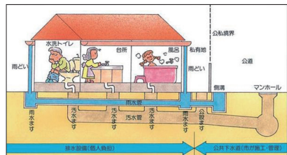
◀下水を運ぶ方式には、汚水と雨水を1本の管で運ぶ合流式と、汚水と雨水を別々の管で運ぶ分流式があり、市では分流式を採用しています。
