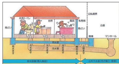
◀下水を運ぶ方式には、汚水と雨水を1本の管で運ぶ合流式と、汚水と雨水を別々の管で運ぶ分流水式があり、市では分流水式を採用しています。
